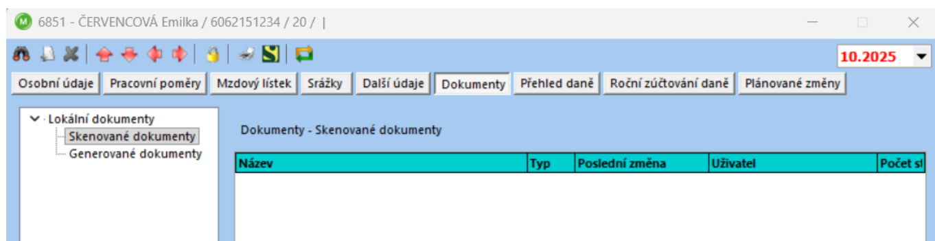
Obrázek 63: Záložka Dokumety
