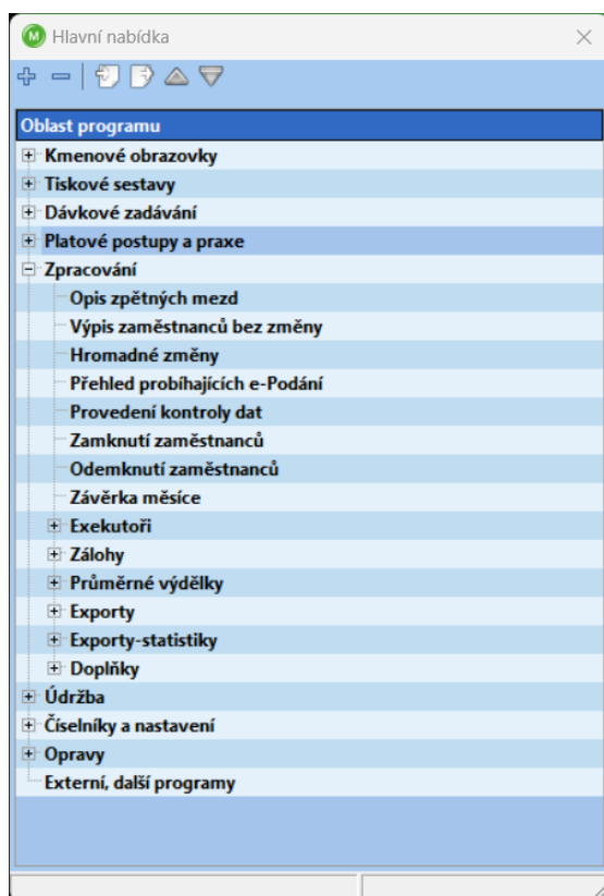
Obrázek 94: Zpracování
