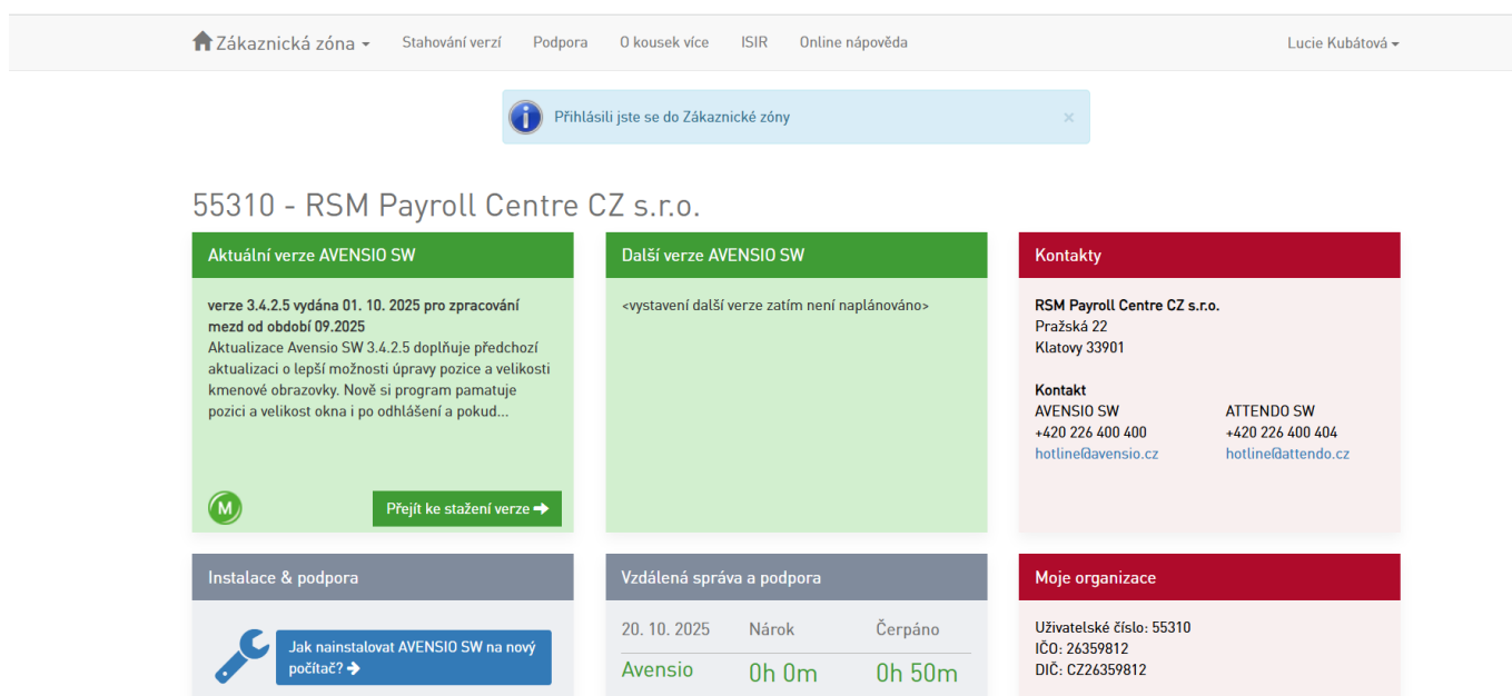
Obrázek 2: Zákaznická zóna
