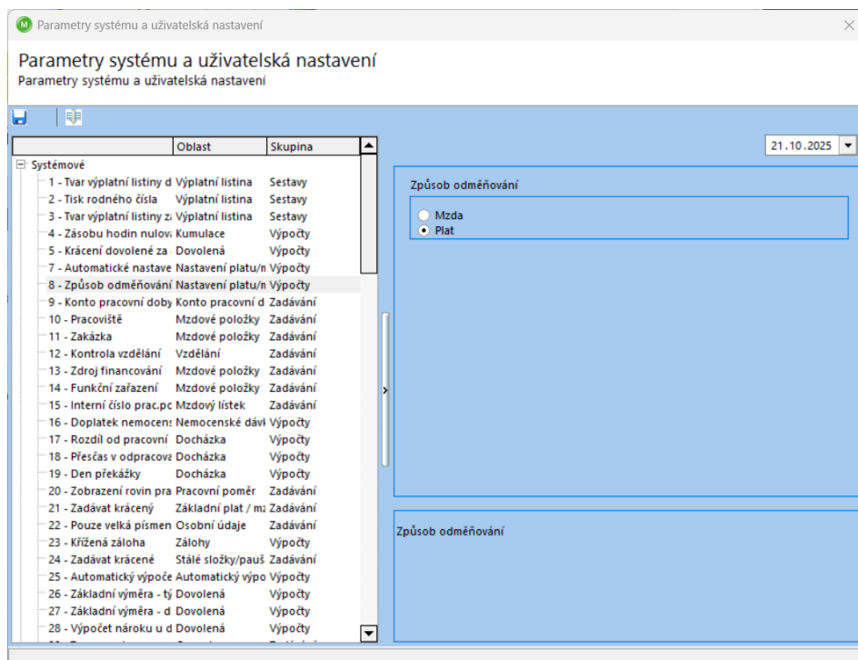
Obrázek 11: Parametry
