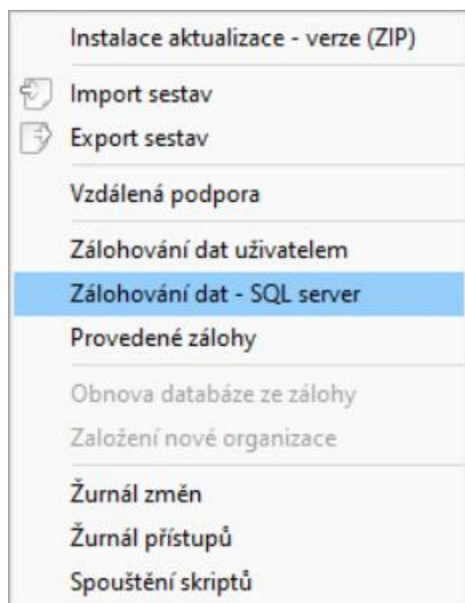
Obrázek 9: Záložka Údržba
