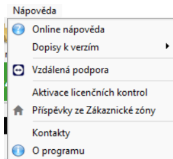
Obrázek 10: Záložka Náповěda
