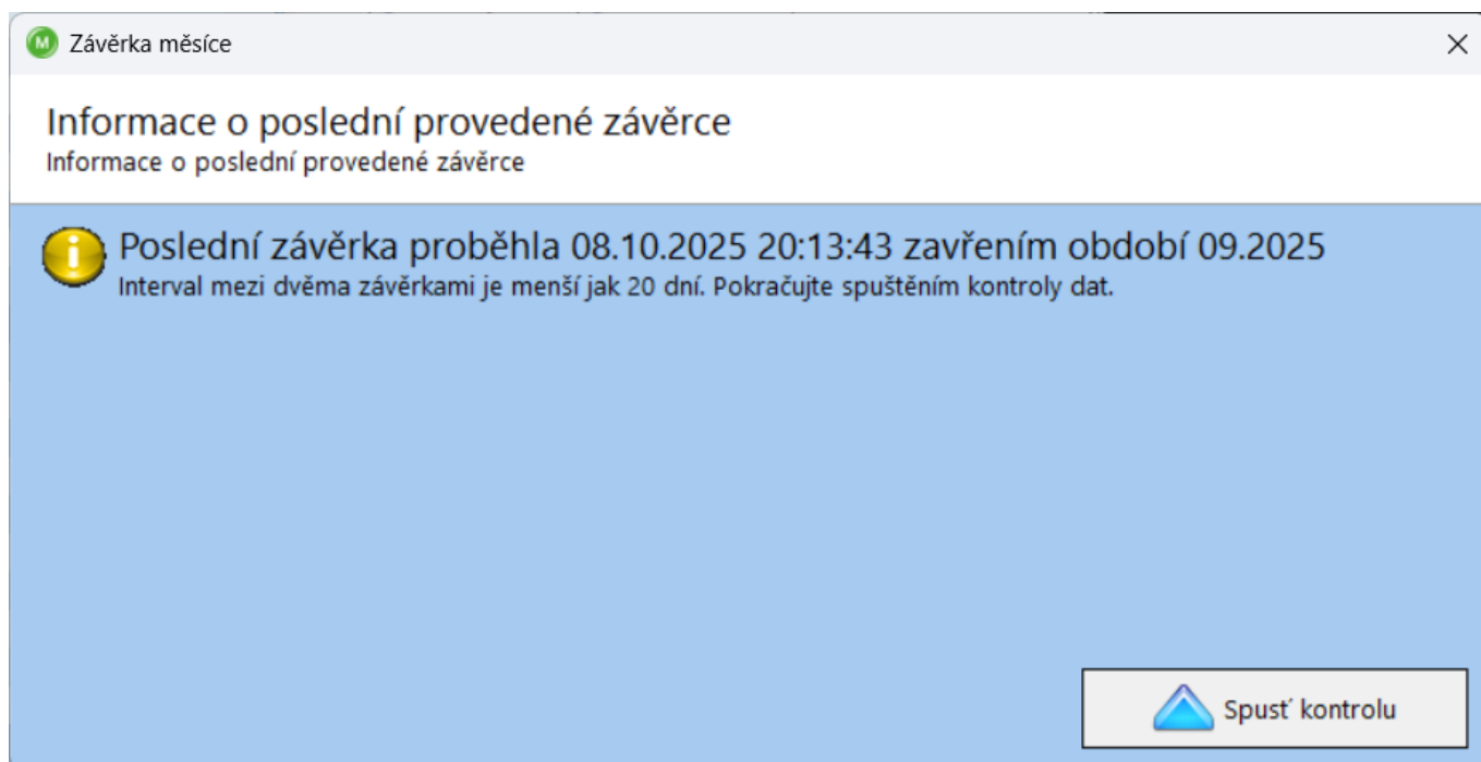
Obrázek 96: Závěrka měsíce
